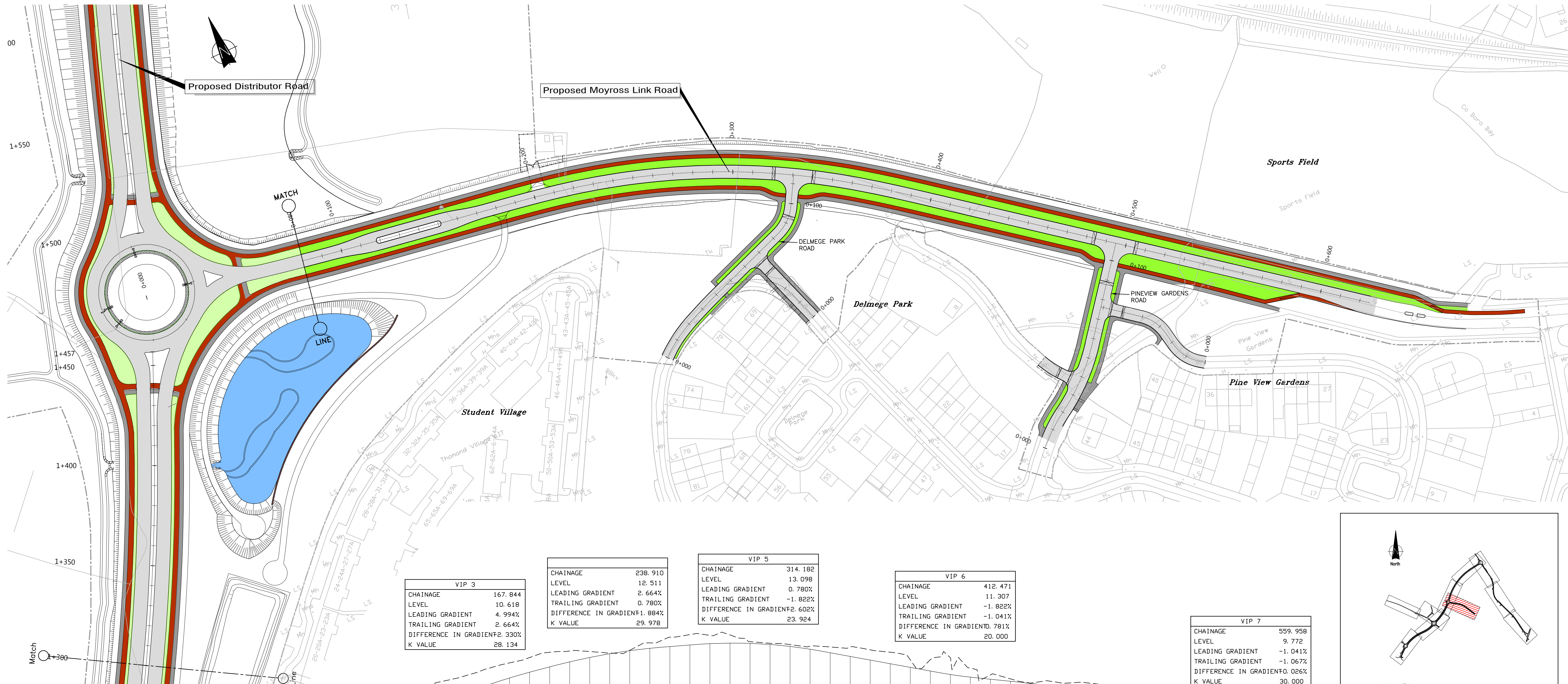
PLAN CH 0+000 - CH 0+600 SCALE 1:1000
