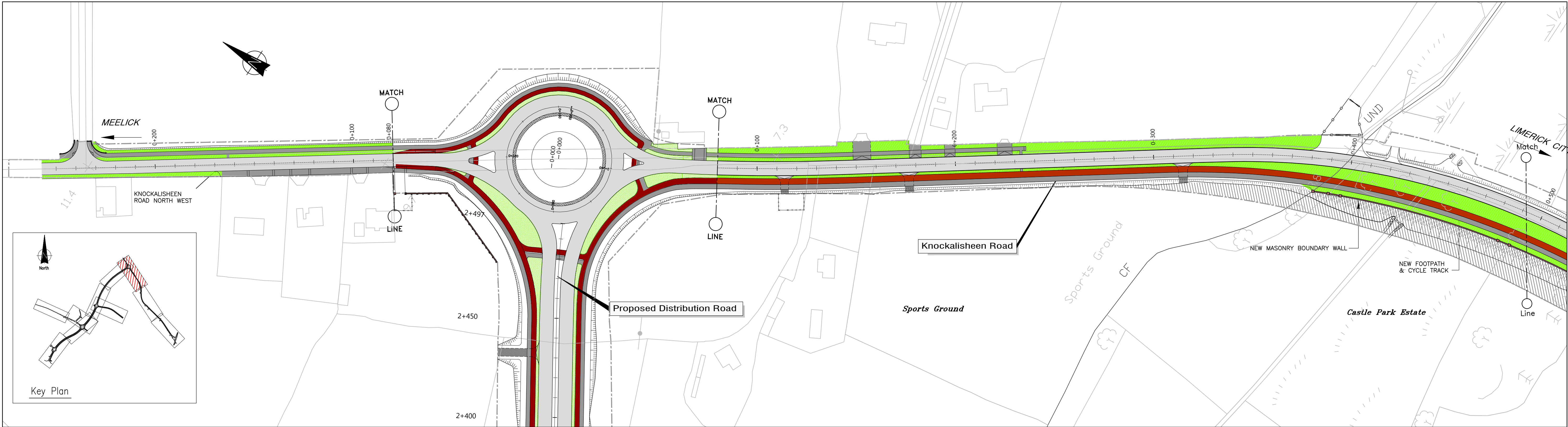
PLAN CH 0+000 - CH 0+500 SCALE 1:1000
